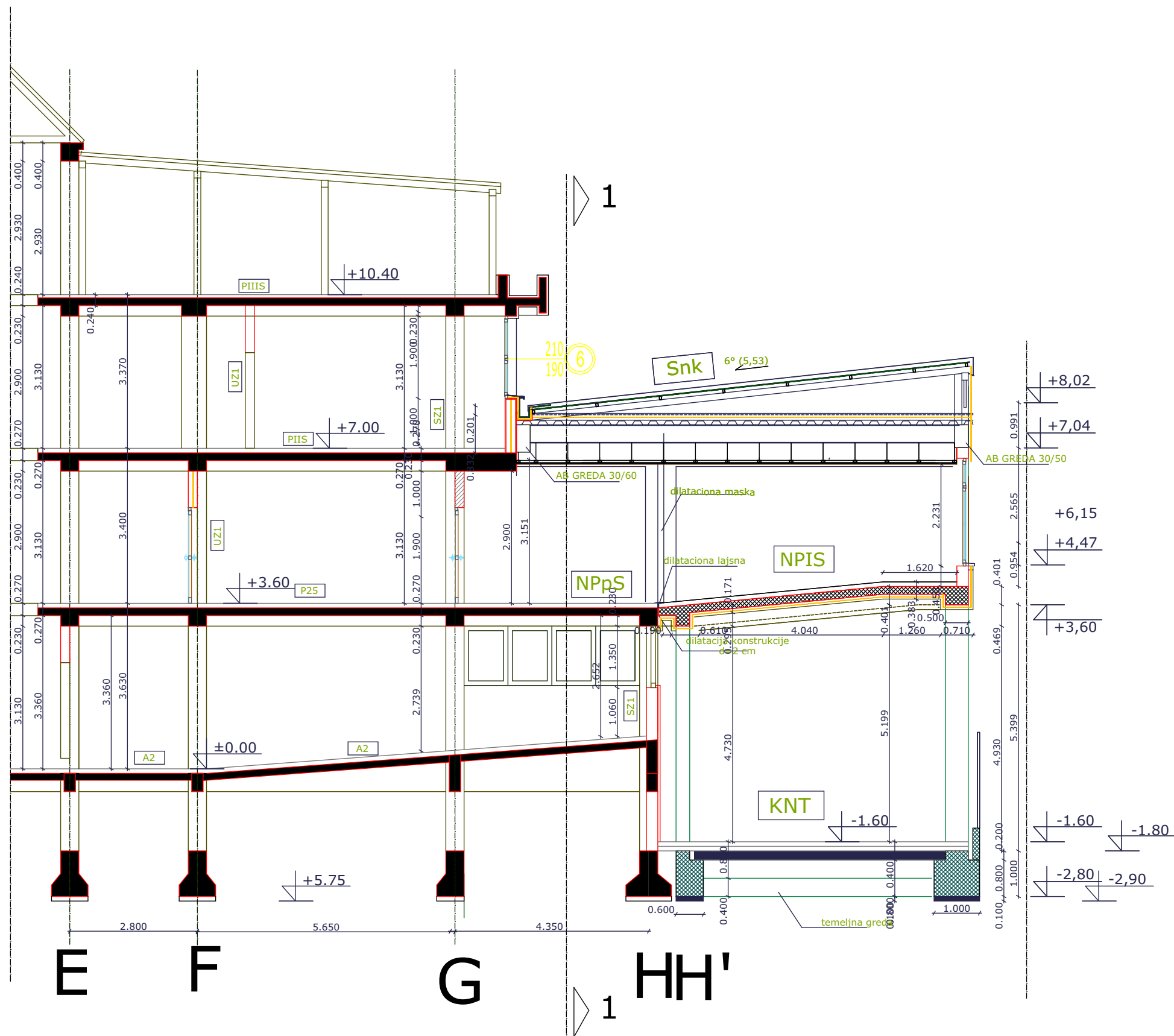
Presek A-A novo stanje R=1:100
